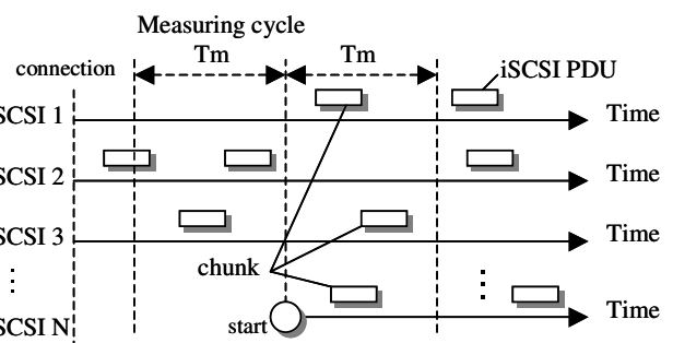
図 9: スループット G の計測; 固定値の計測時間 T_m 中にカウントされる iSCSI PDU 数の合計を不定サイズのチャンクと定義してスループット G を算出する。 ( G = 通過した iSCSI PDU 数/ T_m )
